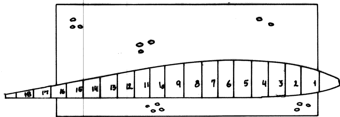
skæreskabeloner vist påsat skum
